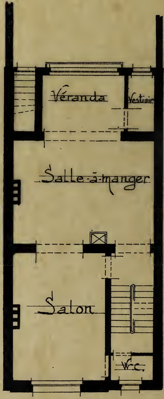
Bel Etage
